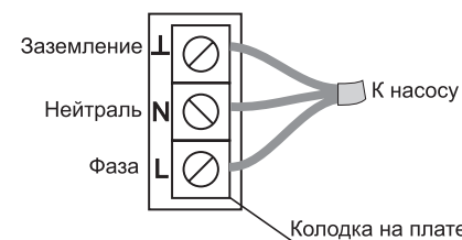
Рис.5 Подключение циркуляционного насоса
