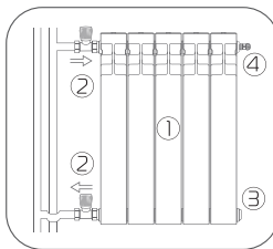
боковое (двухтрубная система отопления)
