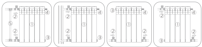
рис. 2 1 - радиатор; 2 - запорно-регулирующий вентиль + переходная гайка; 3 - переходная гайка + заглушка; 4 - переходная гайка + воздухоотводчик; 5 - байпас.
