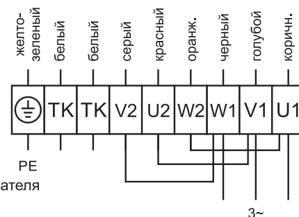
Схема подключения №8
