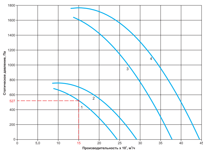
Аэродинамические характеристики вентиляторов РОКС-ВКРС-8,0-ДУ, РОКС-ВКРФ-8,0-ДУ
