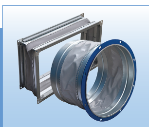
Вставки гибкие
