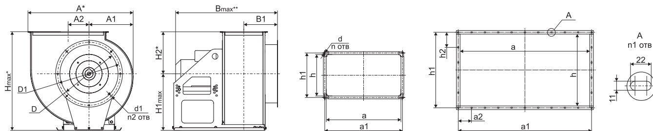
Типоразмер вентиляторов 2,5-8,0
