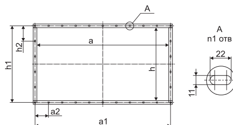
Типоразмер вентиляторов 9,0-12,5
