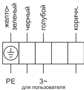
Схема подключения №3
