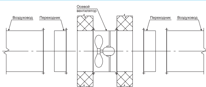
Установка осевого вентилятора с использованием переходников для соединения с воздуховодами
