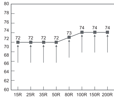
График эффективности теплообмена
