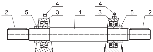
Рисунок 1. Подшипниковая опора
