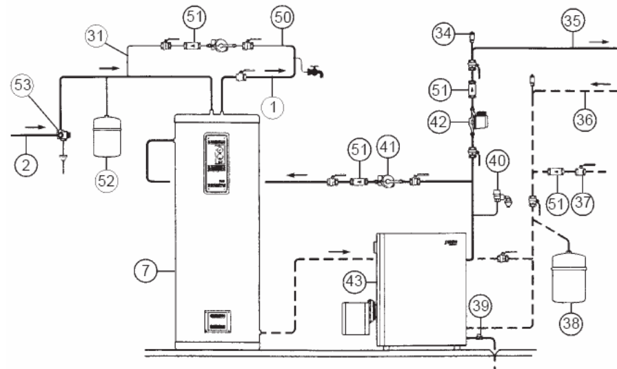
Автономный котел с трехпозиционным клапаном
