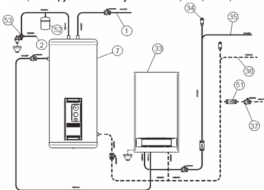
Автономный котел с двумя насосами
