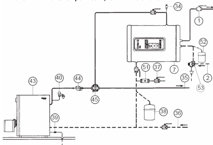
Автономный котел с трехпозиционным клапаном
