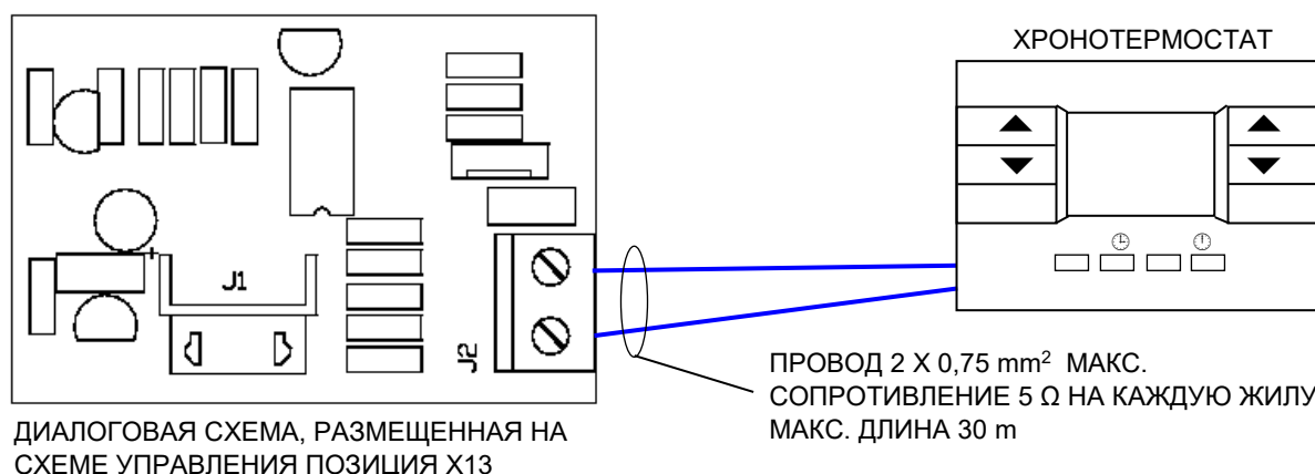
Рисунок 30 – Соединение хронотермостата и диалоговой схемы
