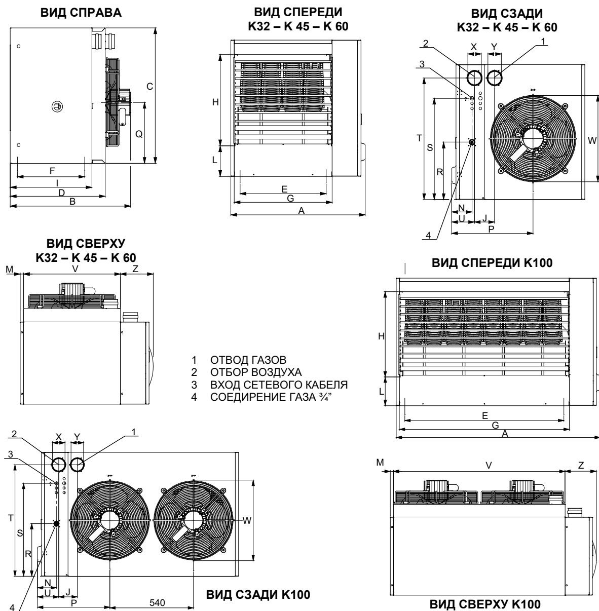
Рисунок 1 – Габариты воздухонагревателей серии К
