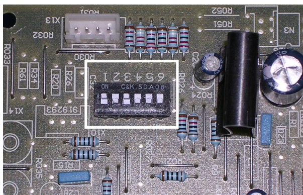
Рисунок 38 – Положение минипереключателей на схеме
