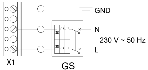
Рисунок 4.1 Подсоединение аппарата к сети электропитания
