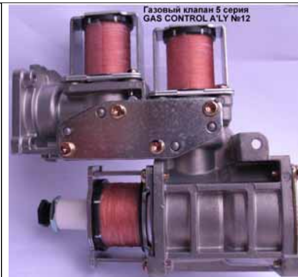
Газовый клапан котла Rinnai 5 сер (Цена 3060 руб)
