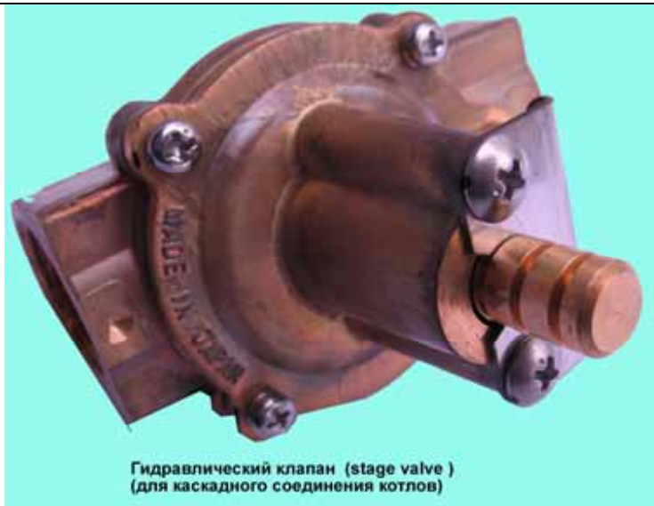
Гидравлический клапан (используется снаружи при каскадном соединении 2-х и более котлов Rinnai) Цена 2700 руб
