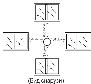
Расположение конца дымохода по отношению к окнам
