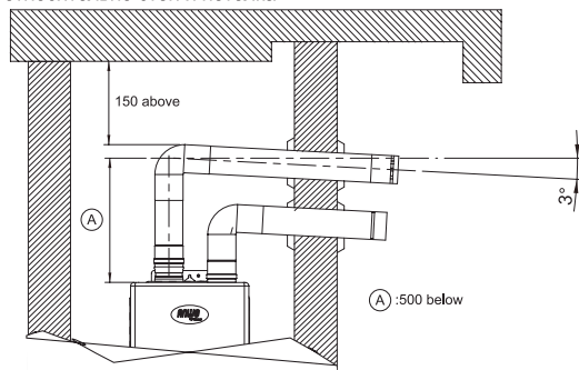
Расположение дымохода относительно стен и потолка (Един измер. мм)
