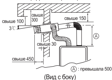
Расположение дымохода относительно стен и потолка. (Един измер. mm)
