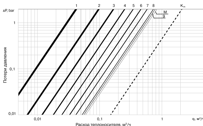
Диаграммы для термостатического клапана без узла нижнего подключения при 2°C
