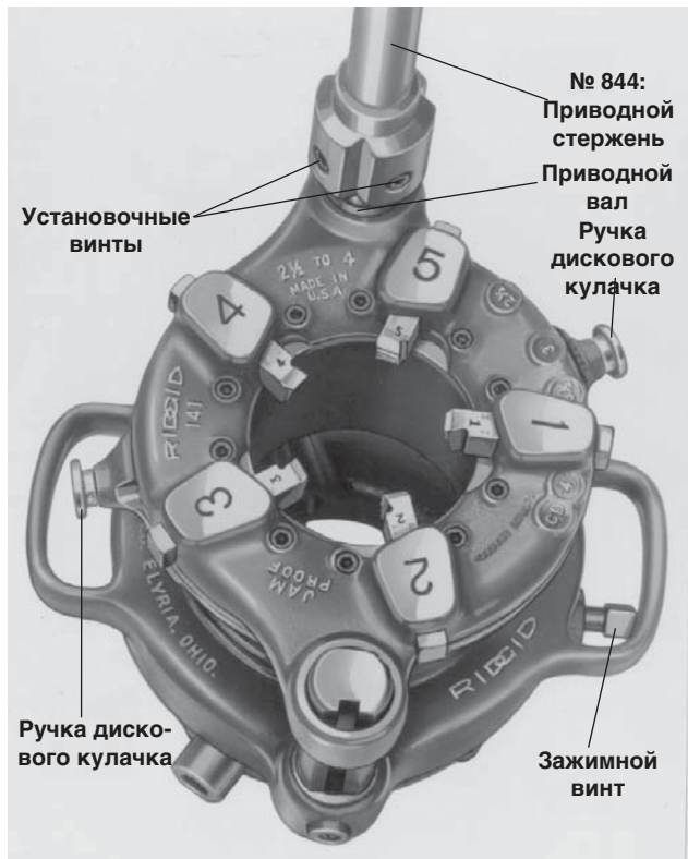
Рисунок 7 – Головка № 141 с зубчатой передачей (то же в случае с головкой № 161)
