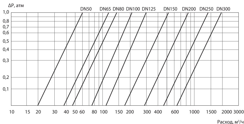
Номограмма потерь давления при полностью открытом затворе регулятора
