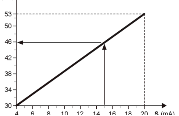
График работы CS зимой при логике со сменой уставки
