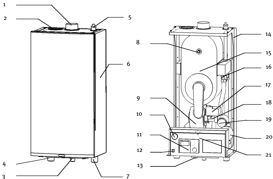
Рис. 3 Общий вид
