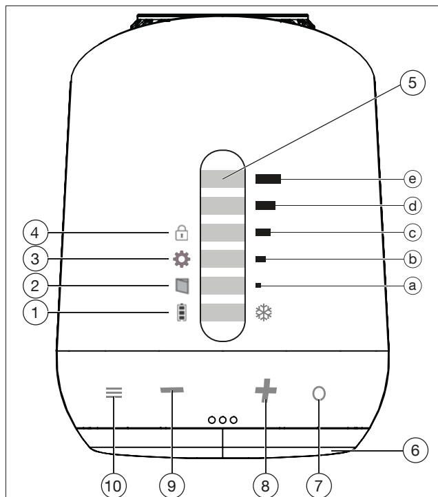
Рис. 1 Элементы управления и индикация
