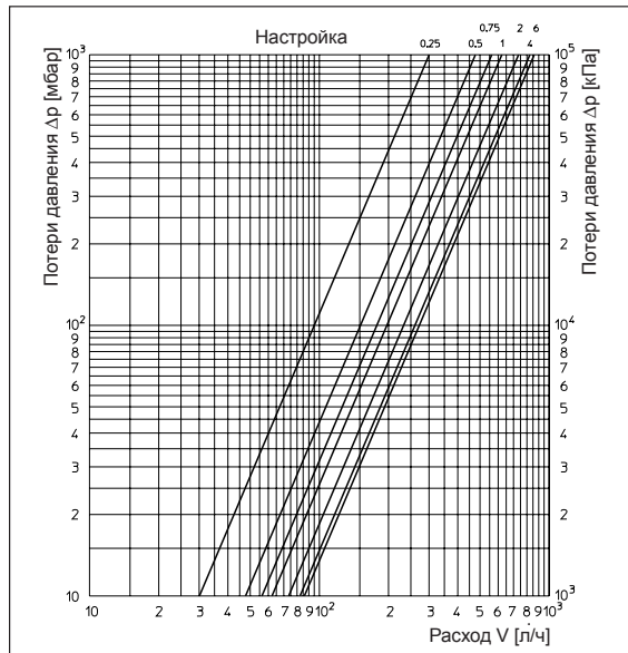
Регулирующ. вставка, 2К Р-отклонен., преднастройка байпаса 1,9 (50%)
