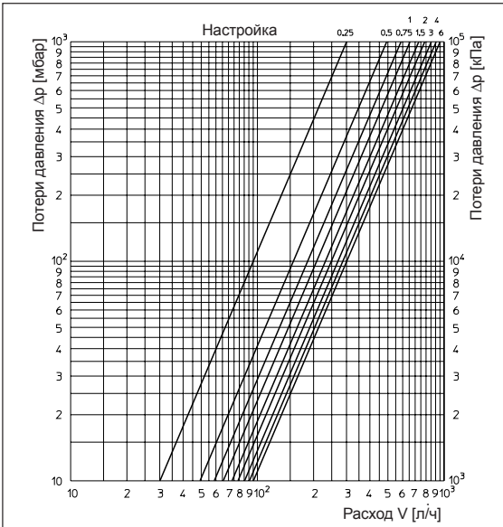
Регулирующ. вставка, 2К Р-отклонен., преднастройка байпаса 2,3 (75%)
