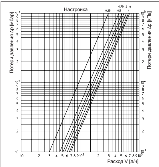
Регулирующ. вставка, 2К Р-отклонен., преднастройка байпаса 1,4 (25%)
