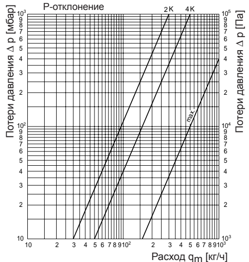
Диаграмма потерь давления „Unibox RTL“
