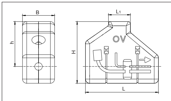
Ду 25
