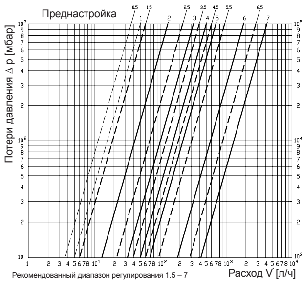
Ду 25
