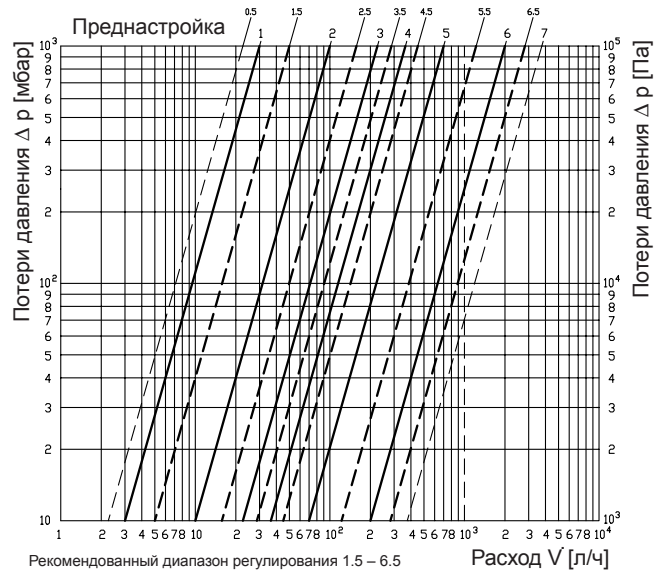
Ду 20
