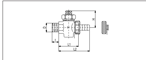
Арт.№ 103 20 03-08 (Ду 10 - DN 25) со штуцером под шланг и колпачком
