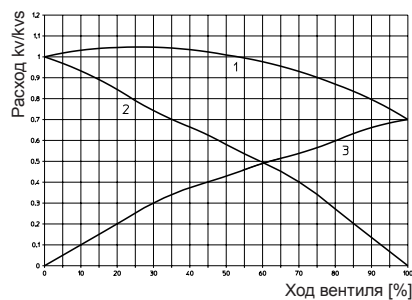
1 Первичн. контур, 2 вторичн. контур, 3 байпас
