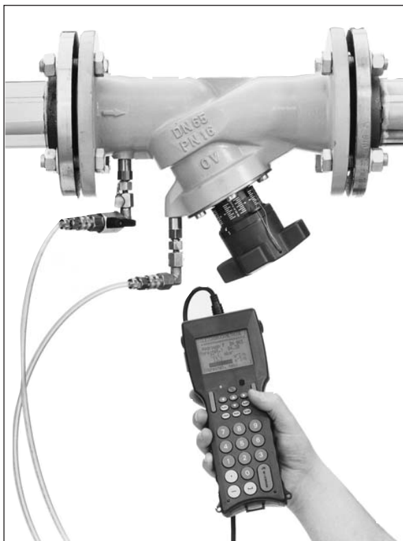
Прибор для измерения расхода Арт. №. 106 91 77 с „Hydrocontrol F” Ду 65
