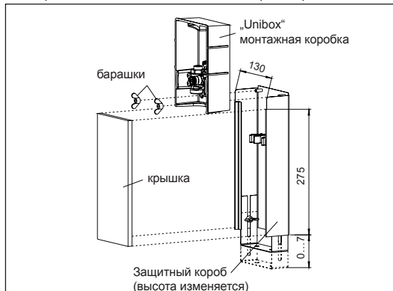
Размеры защитного короба арт. № 102 26 52
