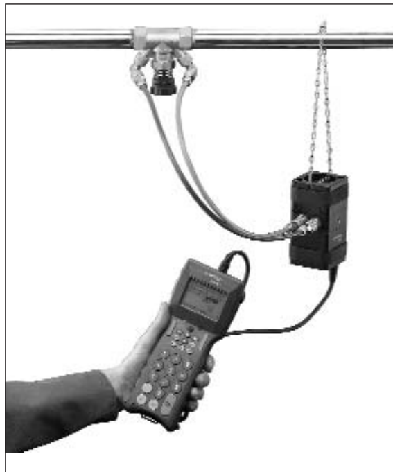
Измерительный компьютер Арт.№ 106 91 77
