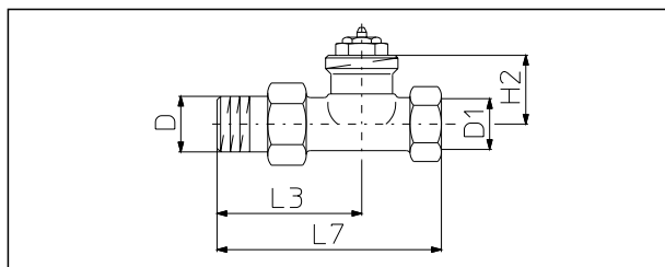
Прходной вентиль
