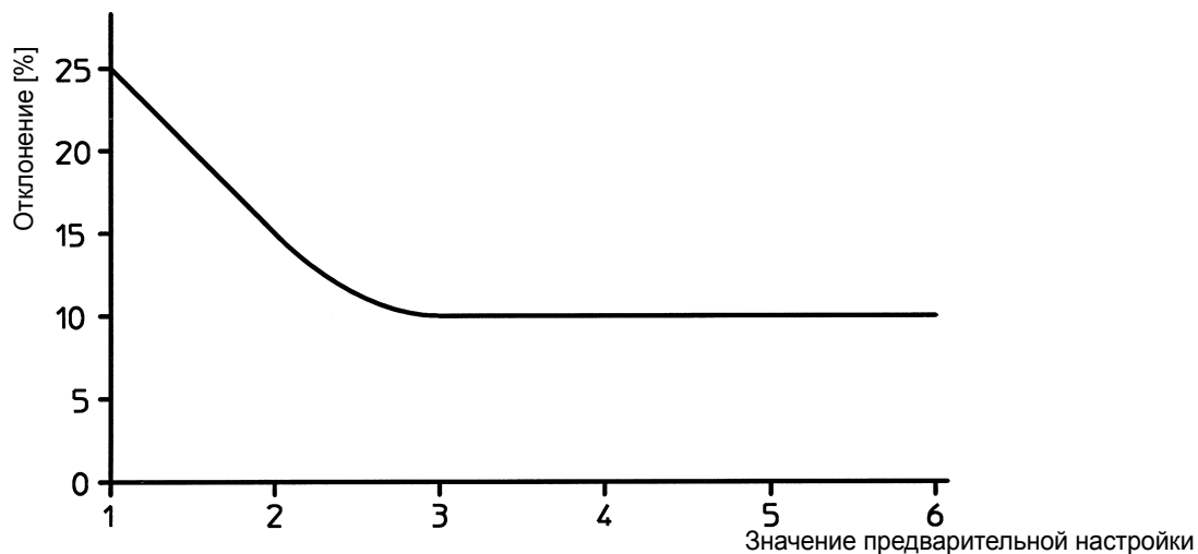
Отклонение расхода в зависимости от преднастройки.
