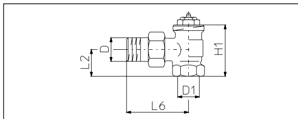
Угловой вентиль
