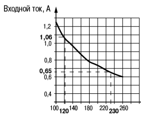
Рисунок 4 - График зависимости входного тока от напряжения питания (без АКБ)
