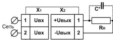
Рисунок 5.1 – Типовая схема подключения блока питания БП02Б – Д1 – 24
