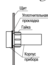
Рисунок 3 – Монтаж прибора щитового крепления
