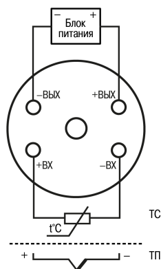
Рисунок 6.2 – Подключение прибора
