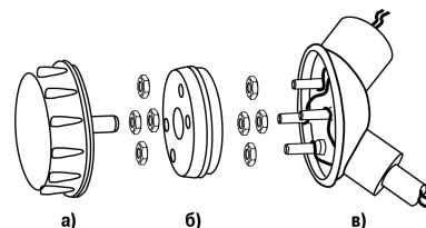
Рисунок 6.3 – Монтаж прибора
