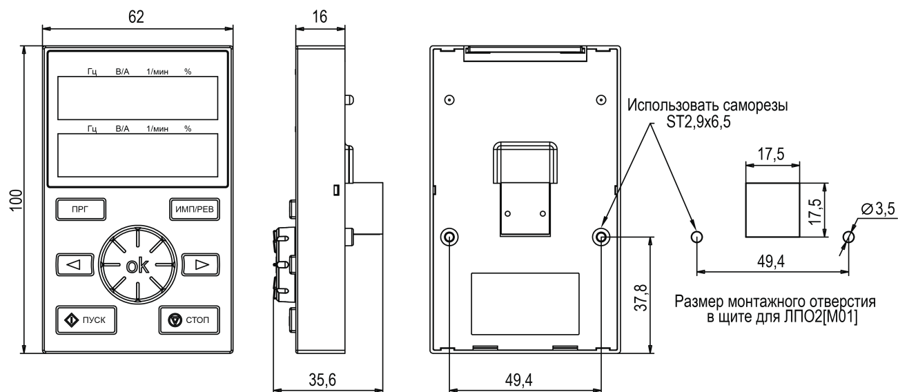
Рисунок 7.9 – Габаритные размеры внешней ЛПО2(М01)
