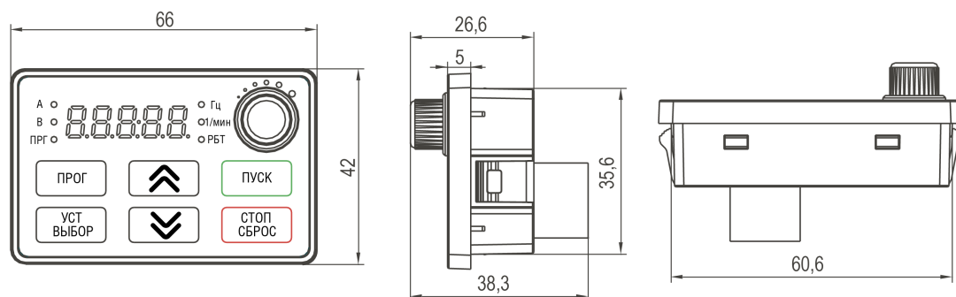
Рисунок 7.8 – Габаритные размеры внешней ЛПО1(М01)
