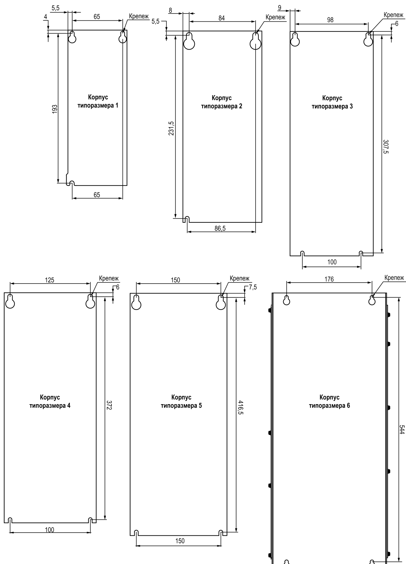
Рисунок 7.7 – Присоединительные размеры
