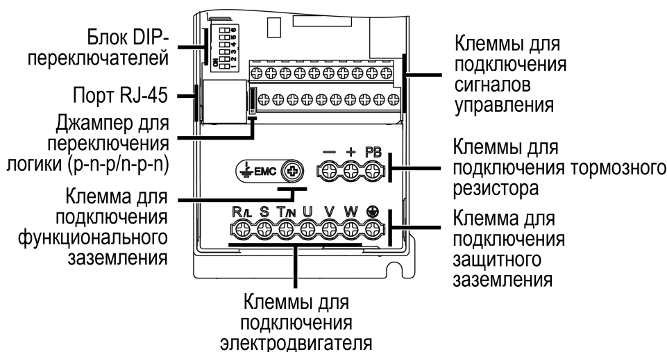
Рисунок 8.3 – Вид на клеммники (крышка снята)
