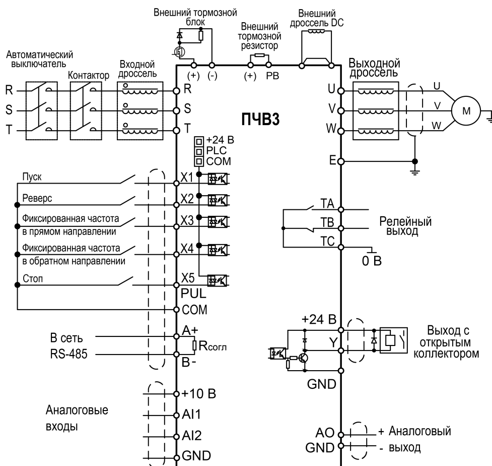
Рисунок 8.4 – Общая схема подключения
