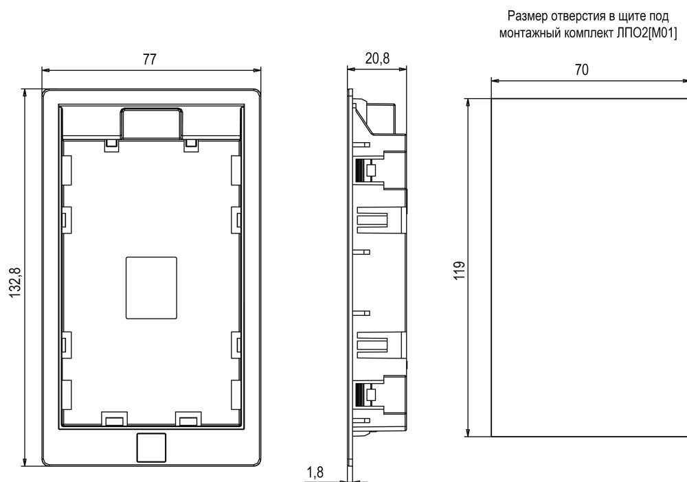
Рисунок 7.10 – Габаритные размеры комплекта для монтажа в щит ЛПО2(М01)
