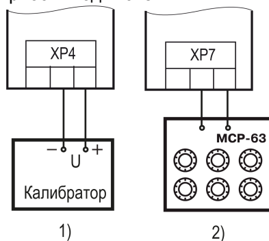
Рисунок Б.1 – Подключение источника эталонного сигнала
