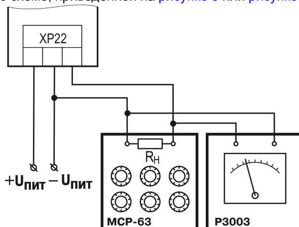
Рисунок Б.3 – Схема подключения к ВЭ для юстировки сигналов типа «4...20 мА» ( R_H < 600 \text{ Ом} )
