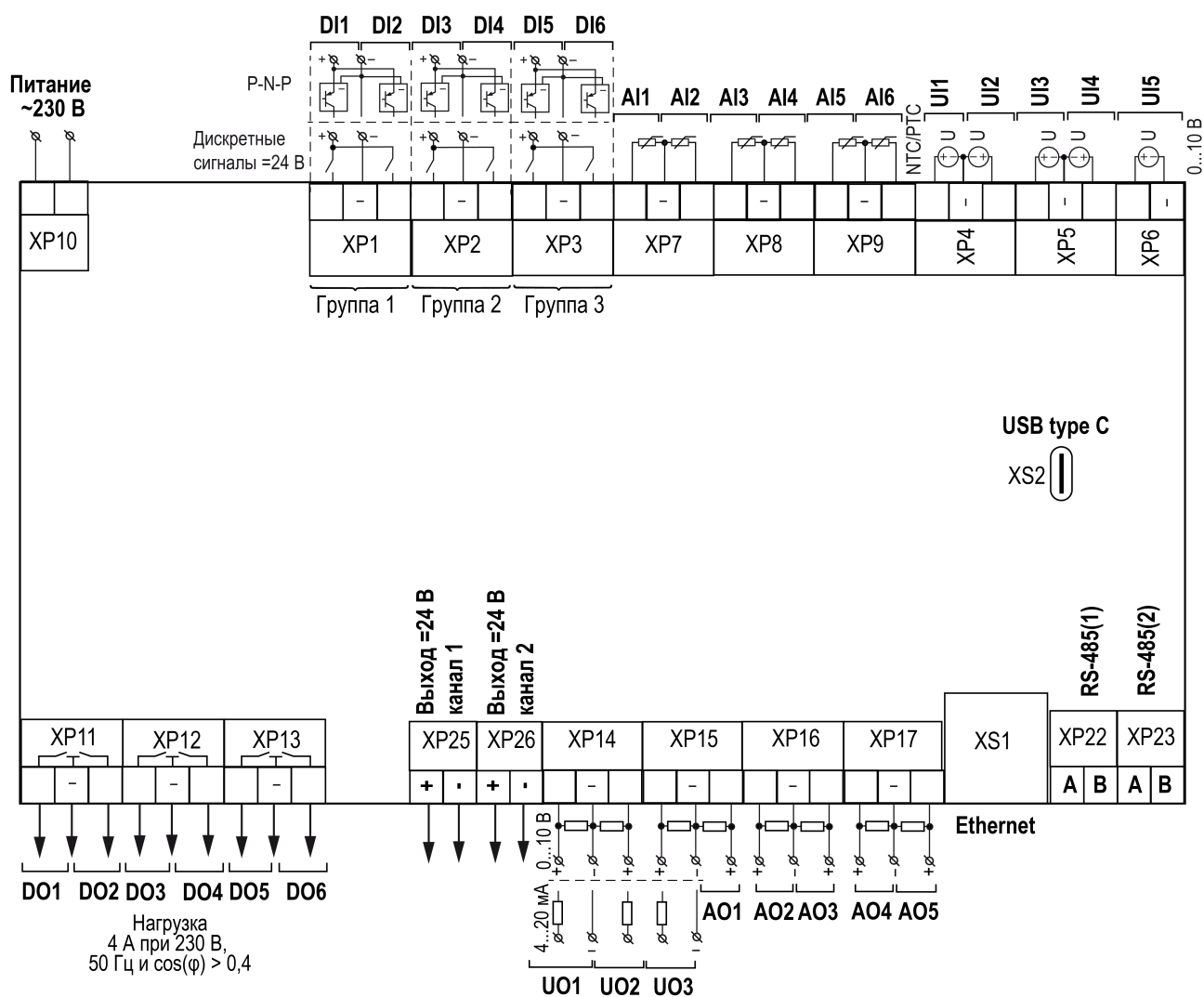
Рисунок 6.2 – Общая схема подключения ОВК–П–230
