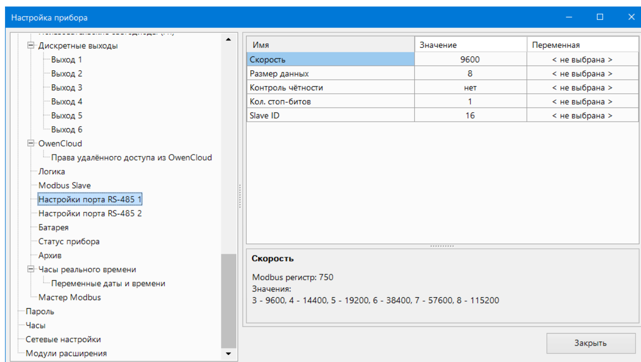
Рисунок 4.20 – Настройки параметров RS-485
