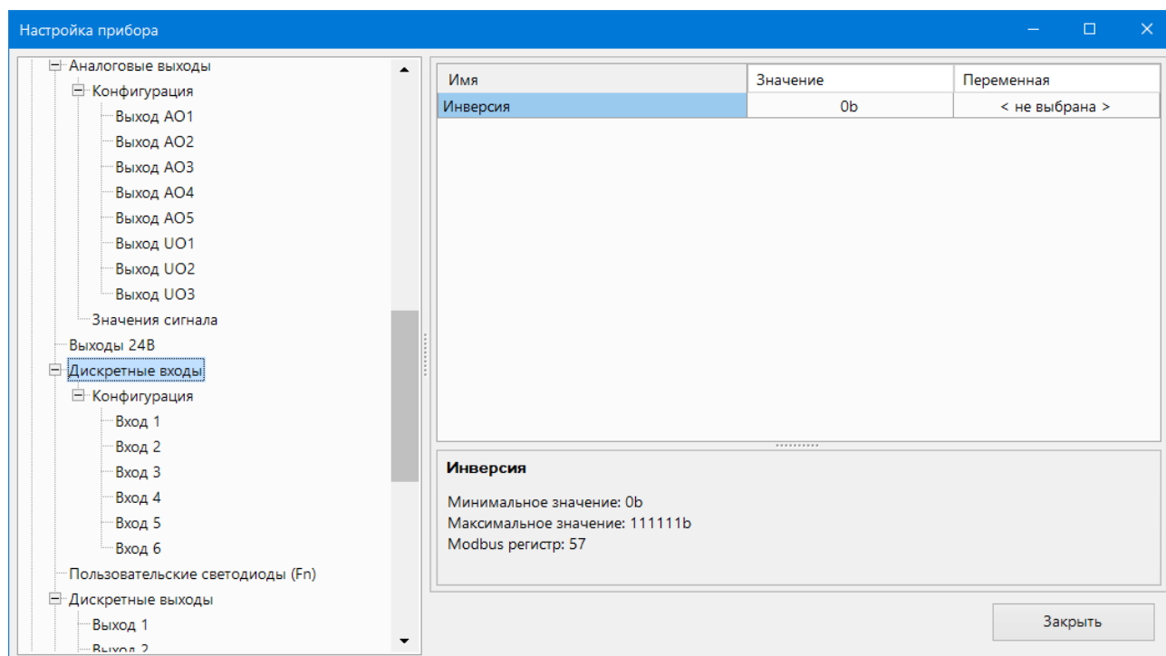
Рисунок 4.7 – Настройка инверсии дискретных входов
