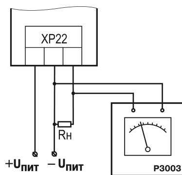
Рисунок Б.4 – Схема подключения нагрузки к ВЭ для юстировки сигналов типа «0...10 В» ( R_n > 600 \text{ Ом} )
