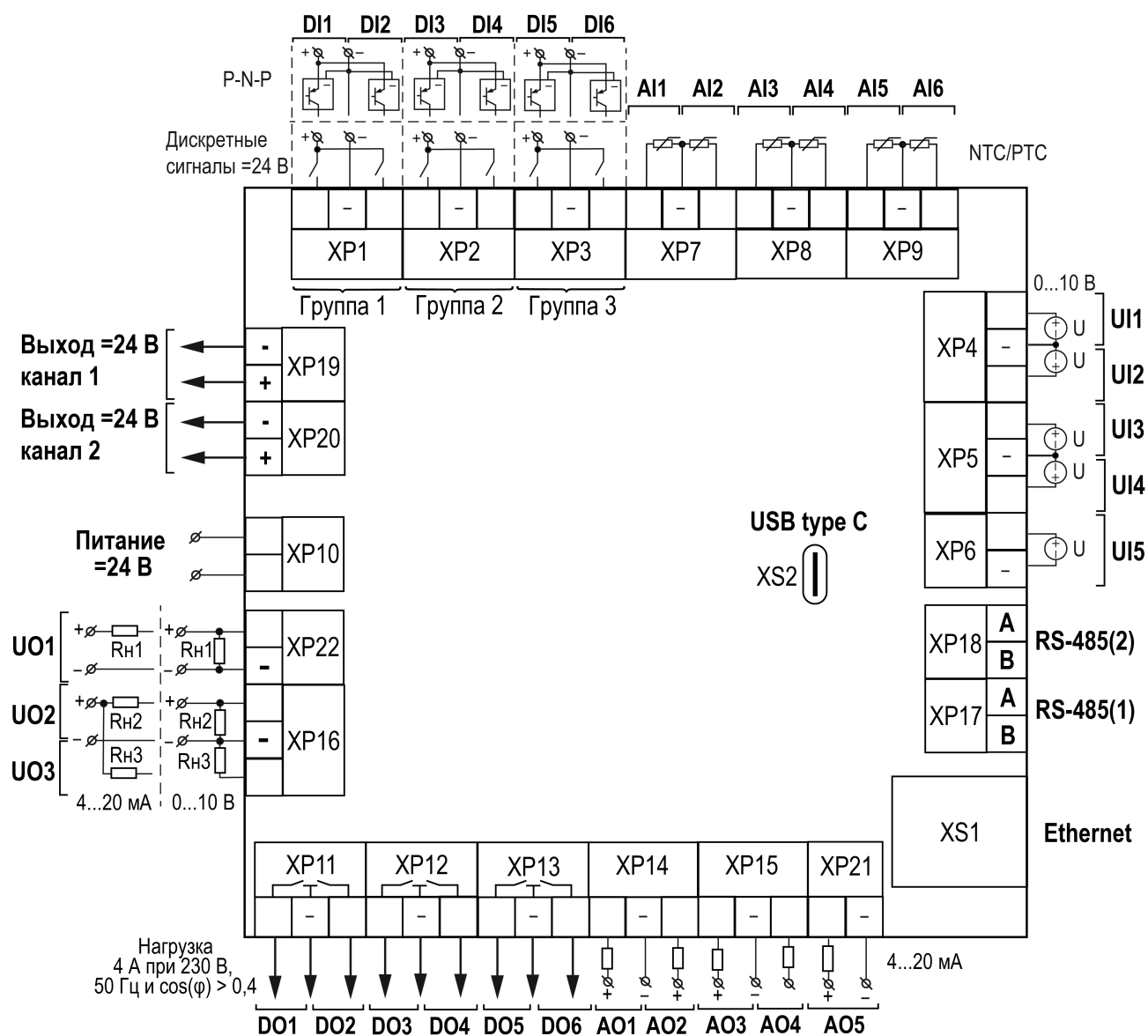
Рисунок 6.1 – Общая схема подключения ОВК-П-24
