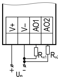
Рисунок 6.21 – Подключение аналогового выхода, находящегося в режиме источника тока
