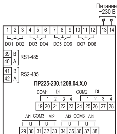
Рисунок А.4 – Расположение контактов для ПР225–230.1208.04.X.0
