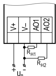
Рисунок 6.22 – Подключение аналогового выхода, находящегося в режиме источника напряжения
