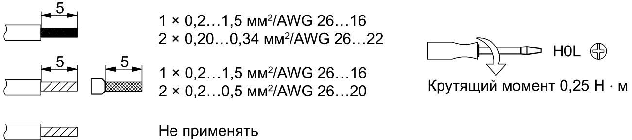
Рисунок 5.1 – Рекомендации для проводов
