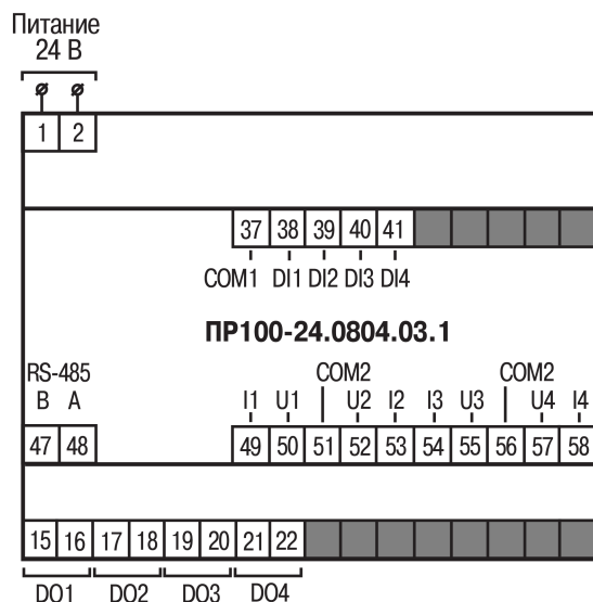
Рисунок А.2 – Расположение контактов для PR100-24.0804.1
