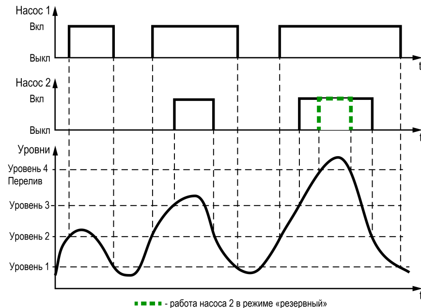
Рисунок 8.1 – Регулирование уровня
