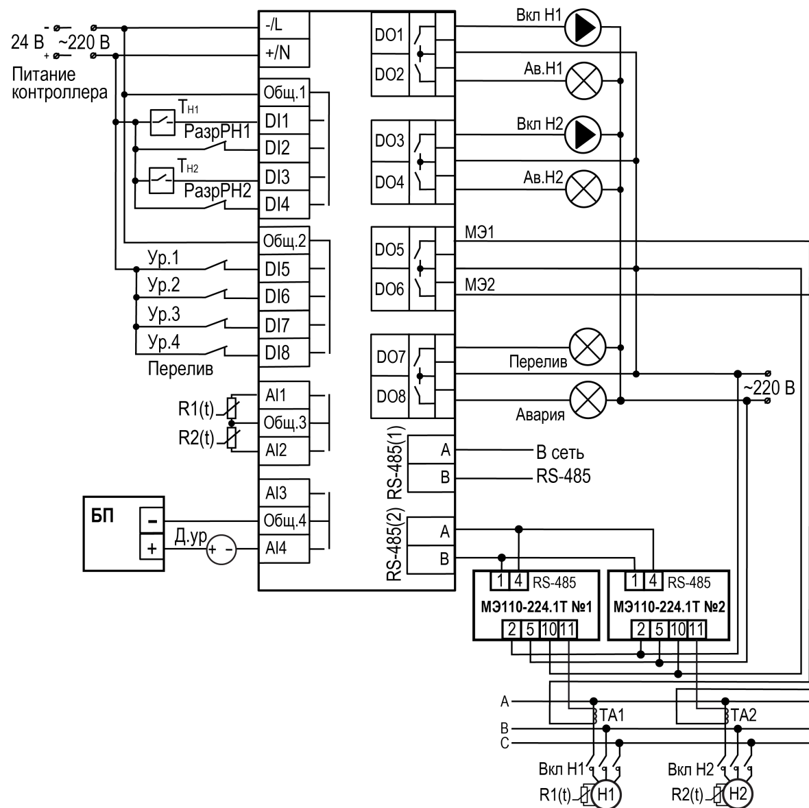
Рисунок 4.4 – Схема подключения СУНА-121.X.09.00
