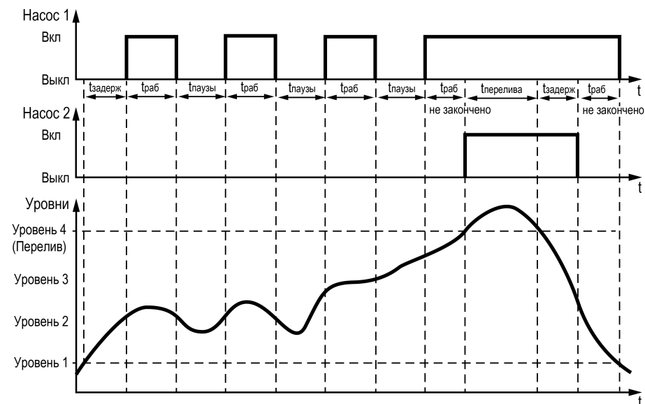
Рисунок 8.4 – Авария дискретных датчиков уровня
