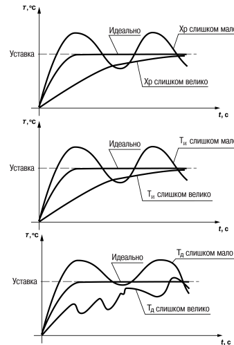
Рисунок Б.1 – Различные виды переходного процесса
