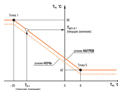
Рисунок 4.6 – Регулирование температуры в контуре по температуре наружного воздуха
