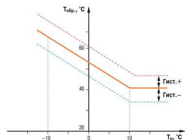
Рисунок 4.7 – График зависимости температуры обратной воды от температуры наружного воздуха
