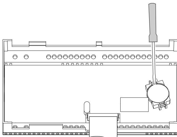
Рисунок 10.2 – Замена батарейки
