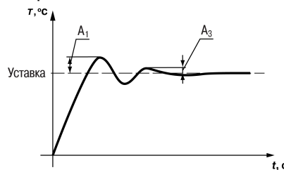
Рисунок Б.2 – График для определения ошибки регулирования
