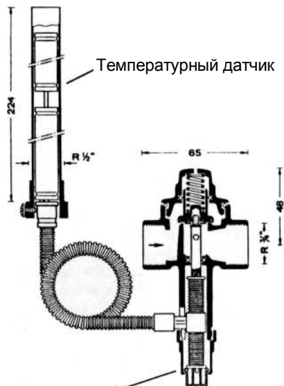
Сильфонная система
