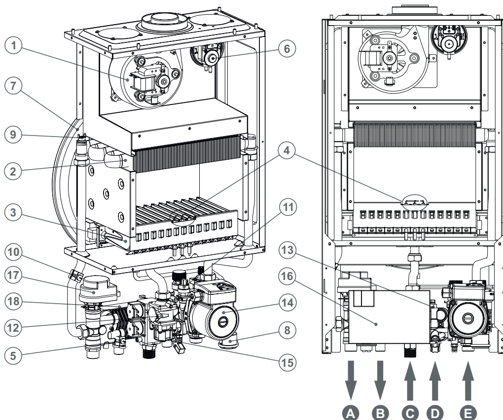
Рисунок 4.2. Общий вид котла ОЧАГ-28Е
