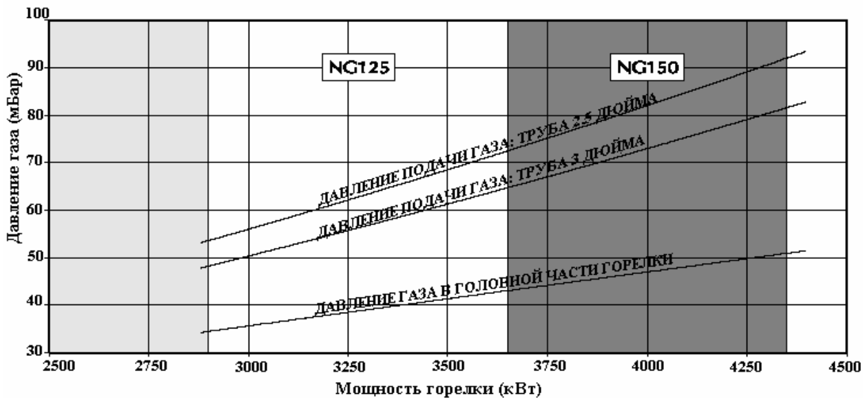
График составлен для природного газа с теплотворной способностью 38.56 Мj/m3
