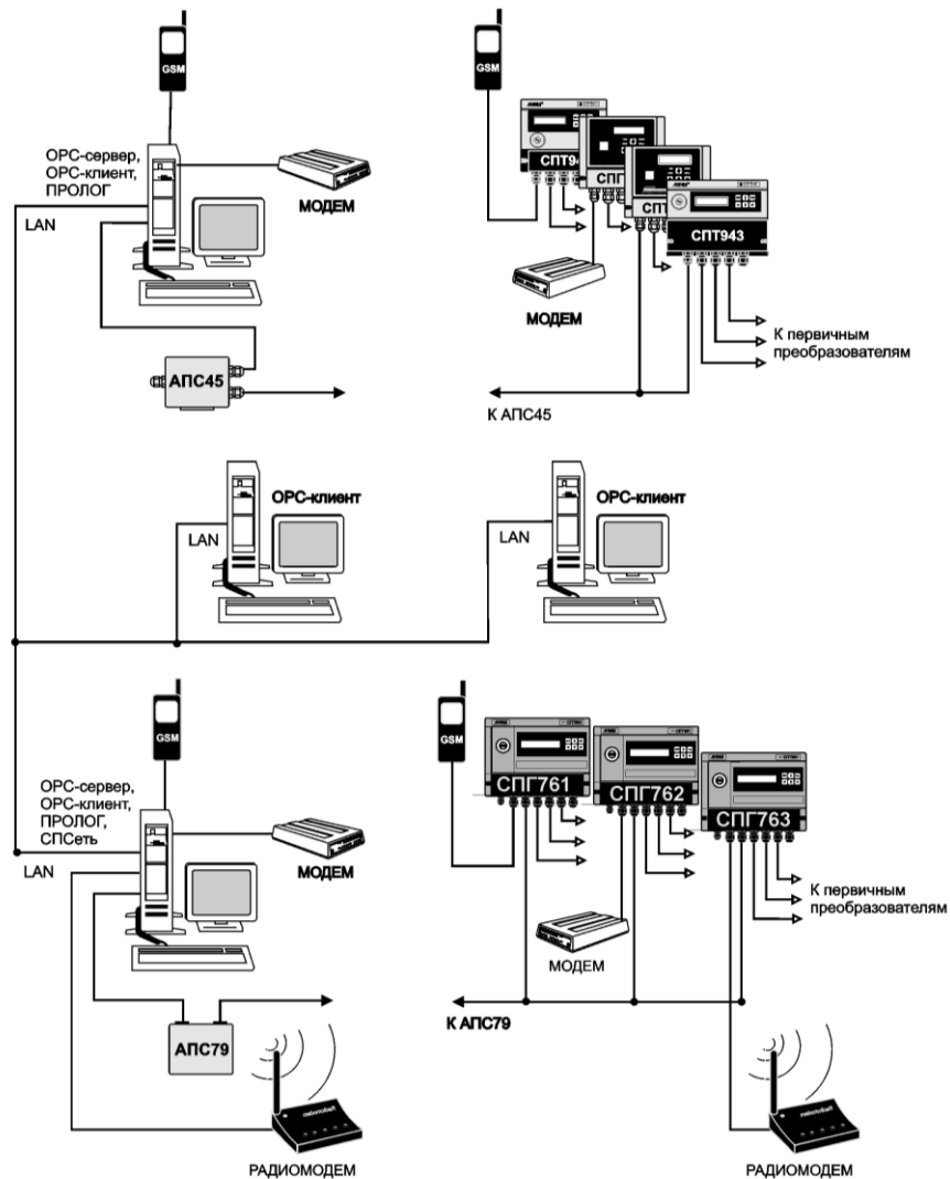
Рисунок 2.2 – Система информационного обеспечения учета энергоресурсов
