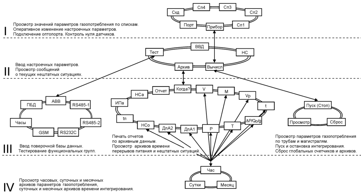
Рисунок 5.1 – Структура меню
