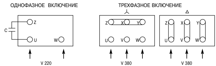
рис. 1 Подключение к электросети
