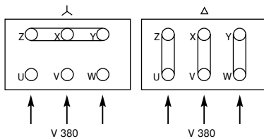
рис. 2 Подключение к электросети
