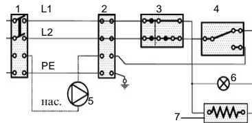
Рис. 3 Электросхема
