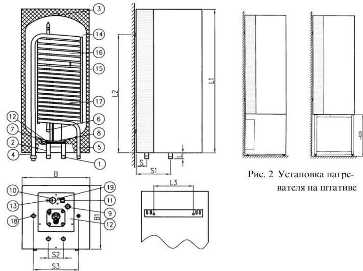
Рис. 1 Конструкция нагревателя
