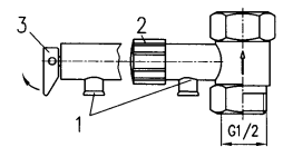
Рис. 4 Предохранительный клапан
