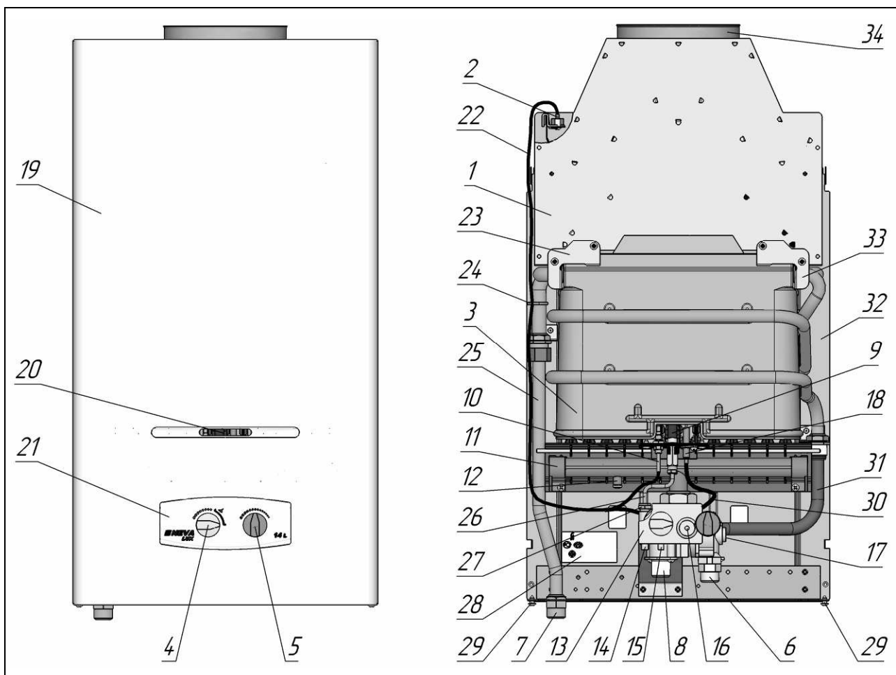
Рисунок 1. Вид аппарата
